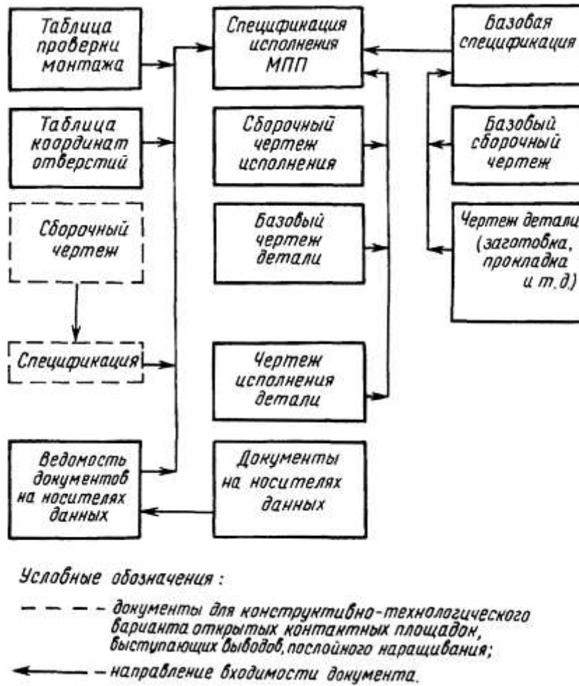
Рисунок 1 - Пример построения комплекта конструкторских документов для МПП
